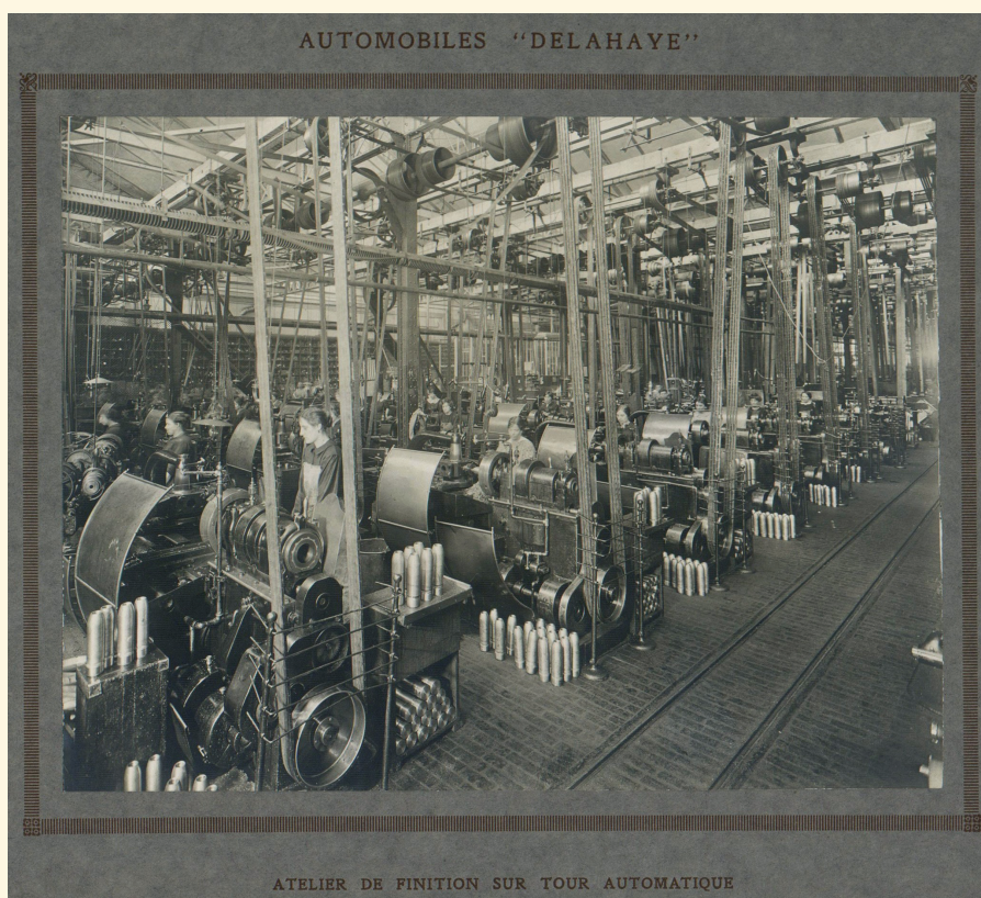
Atelier de finition des obus sur tour automatique, album photographique « Société automobiles Delahaye », ANMT, 2014 39 2, Pièces isolées iconographiques.
